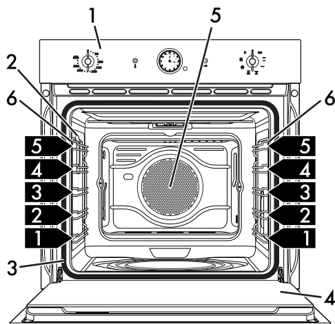
Pyrolytisk modell
